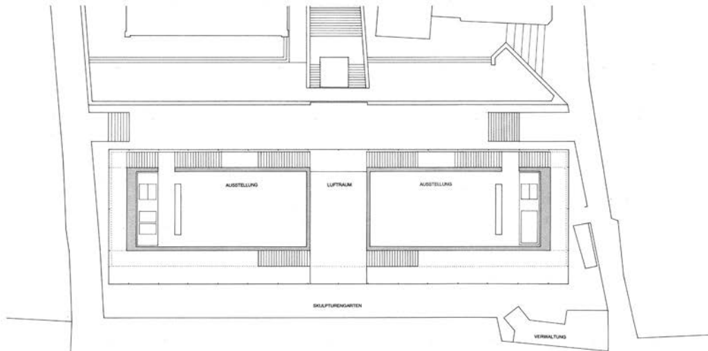
1. OBERGESCHOSS + 288,25
