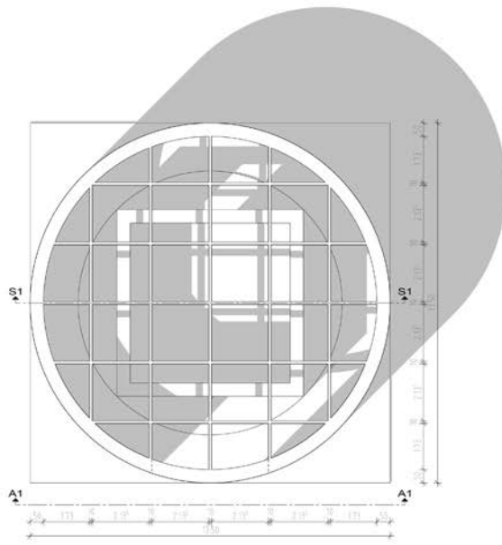
DACHAUFSICHT
